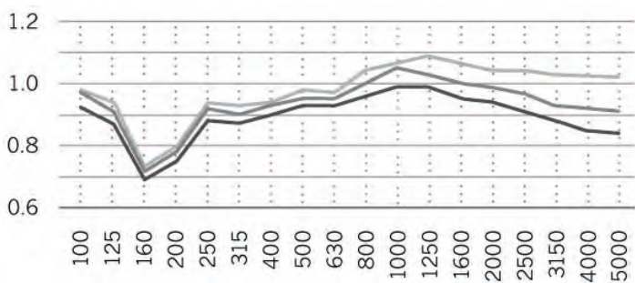
Schallabsorptionsgrad / Terzmittelfrequenz (Hz)
